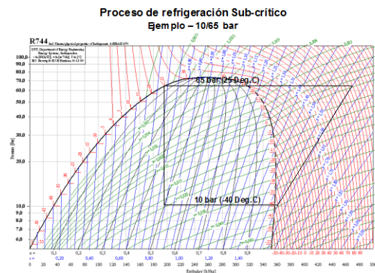
Figura 3. Diagrama LogP-h para circuito subcrítico -40/25^{\circ}\text{C} (10/65 bar)
