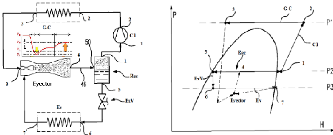
Figura 21. Eyector. Configuración básica del sistema. Representación en diagrama logP-h
