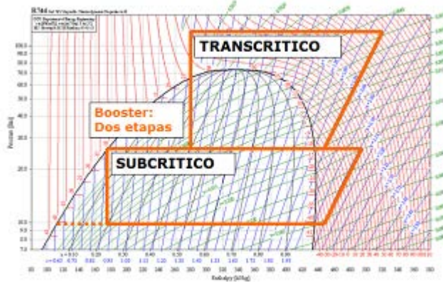
Figura 6. Sistema booster de \text{CO}_2 con dos etapas de compresión
