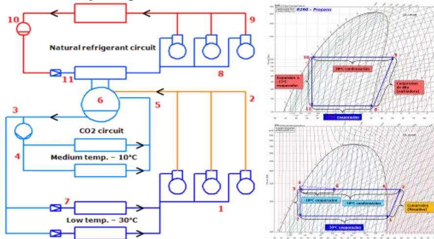
Figura 11. Sistema en cascada de refrigerantes naturales con CO 2 bombeado para MT y expansión seca BT.
