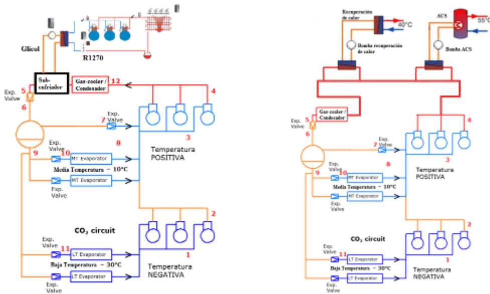
Figura 19. Subenfriador y recuperación de calor y ACS en sistema booster de CO 2
