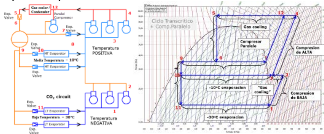
Figura 18. Compresor en paralelo en sistema booster de CO 2
