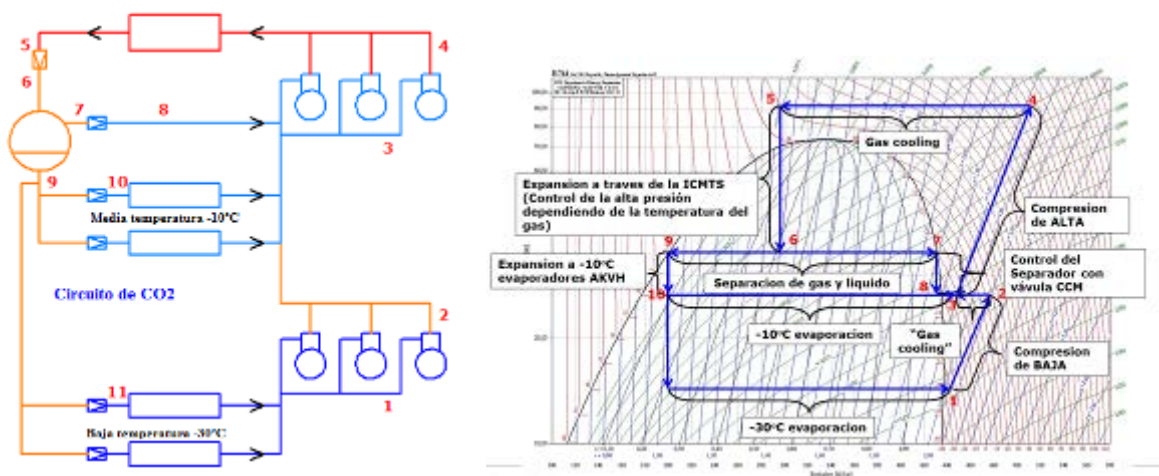
Figura 15. Sistema booster de CO 2 sencillo
