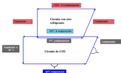
Figura 7. Sistema en cascada de \text{CO}_2 genérico
