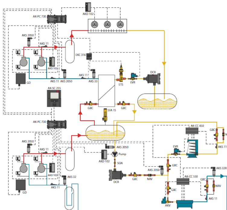
Figura 12. Sistema en cascada de CO 2 bombeado para MT y expansión seca BT con controles.
