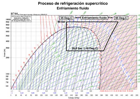
Figura 4. Diagrama LogP-h para circuito transcrito -10/35°C (26,5/90 bar)
