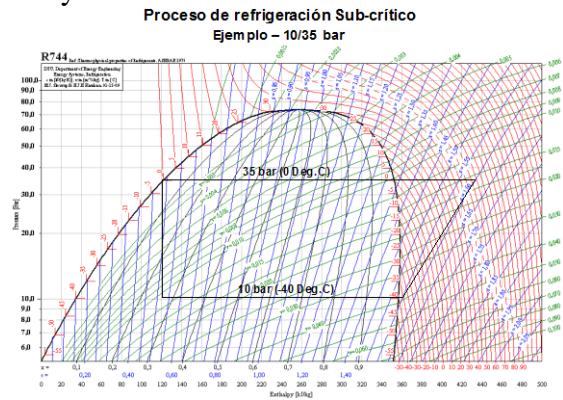
Figura 2. Diagrama LogP-h para circuito subcrítico -40/0^{\circ}\text{C} (10/35 bar)
