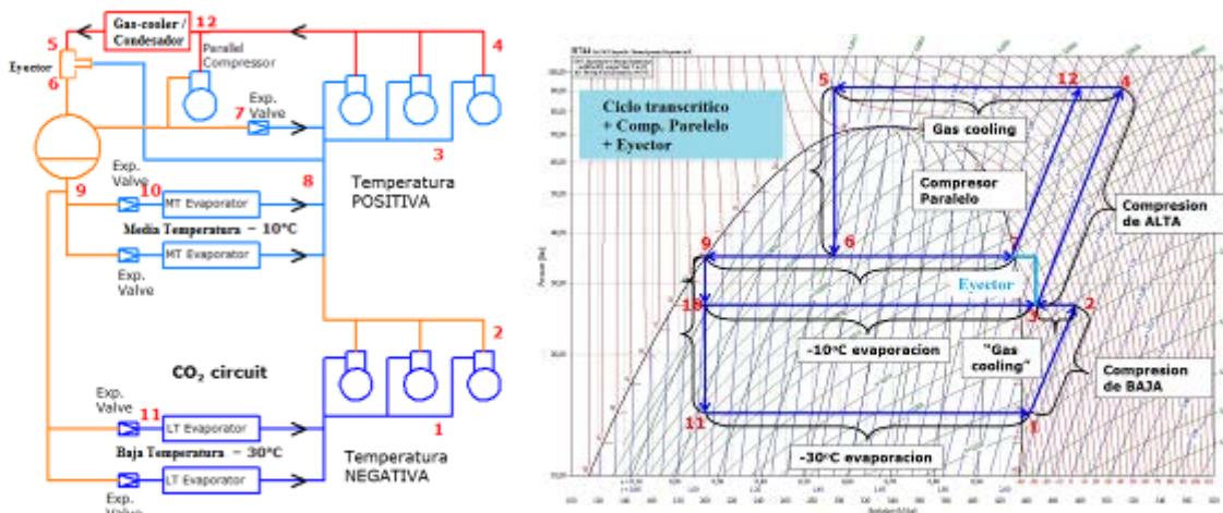
Figura 22. Esquema de sistema booster de CO 2 avanzado con eyector
